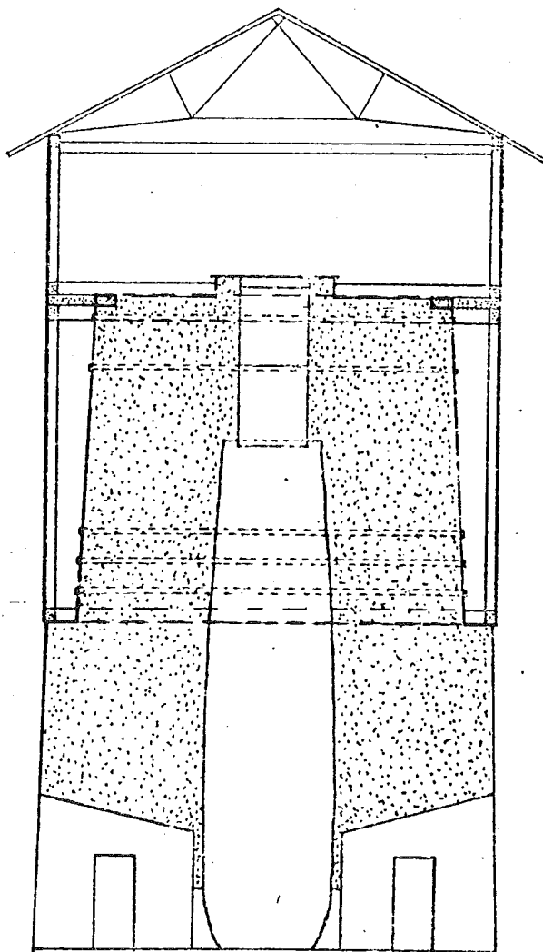
Genomskärning av masugnen i öst-västlig riktning.
